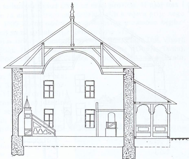
Presjek A—B
