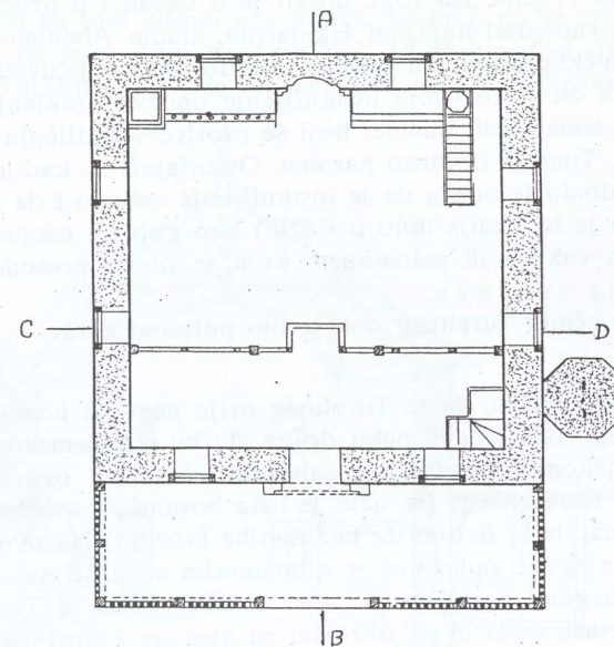
Turalibegova džamija u Tuzli — Osnova 1:200
